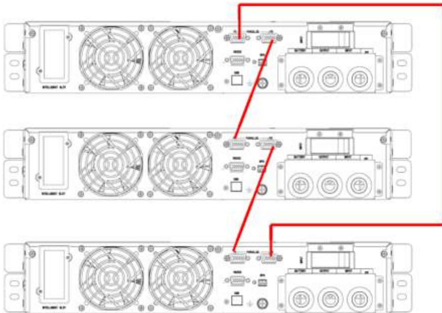
Figura: Sistema de 3 nobreaks em paralelo
